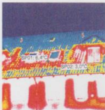
Termografering
