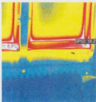
Termografering - vindue
